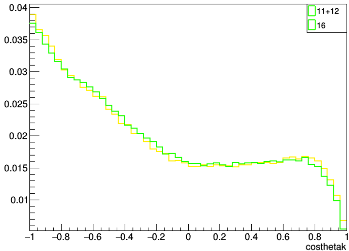
costhetak
