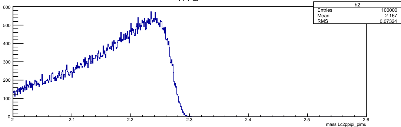
Lc2ppipi_pimu
